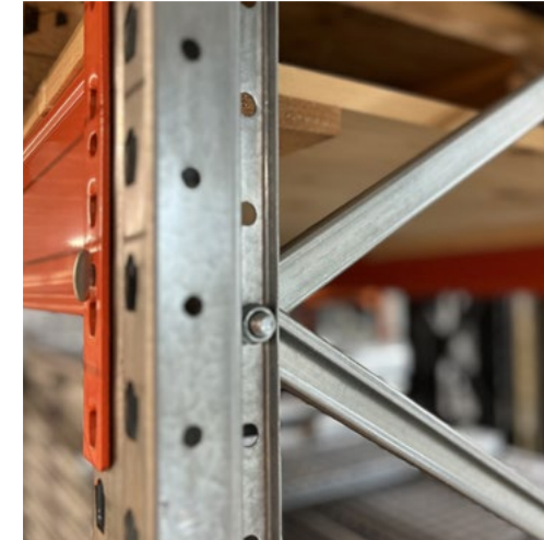
Bevestiging van de schuine schoren in de staander van de palletstelling
